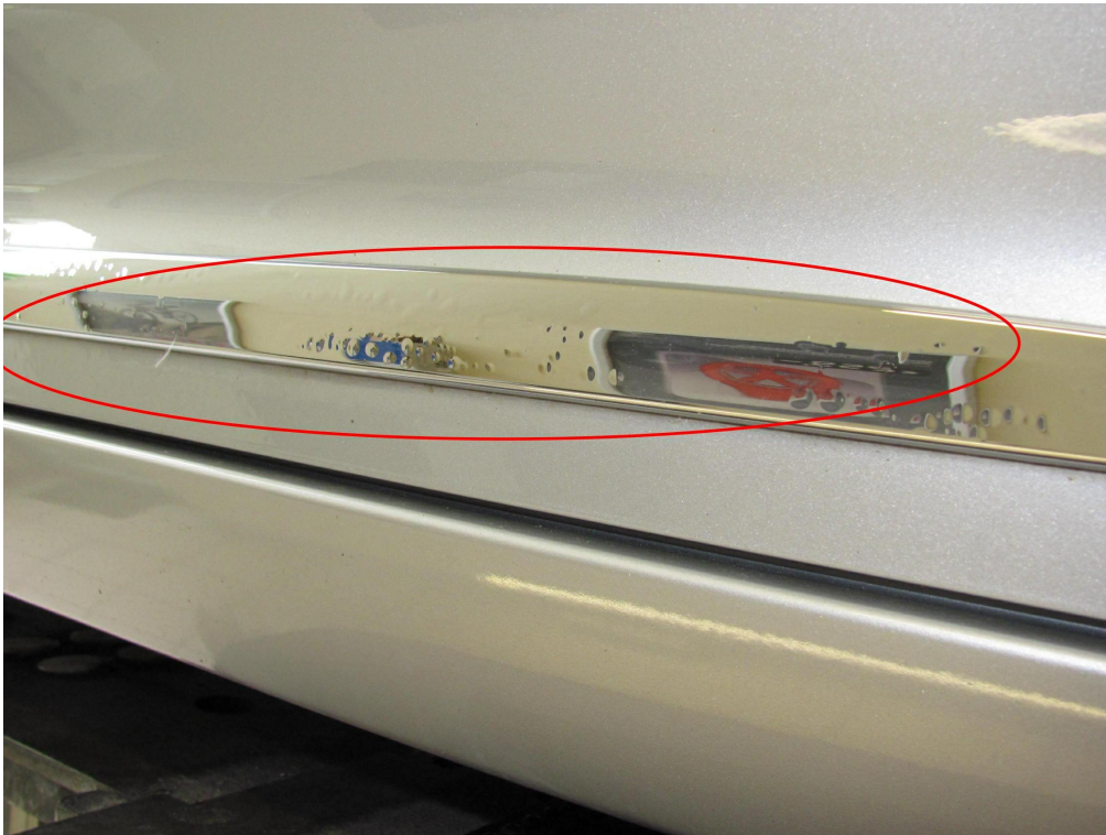
Bild:7 Chromleisten Tür VL,HR u. VR oxidiert
